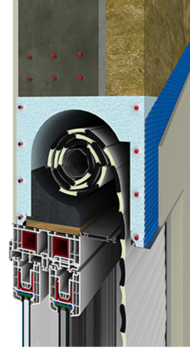
Lento Panjur
